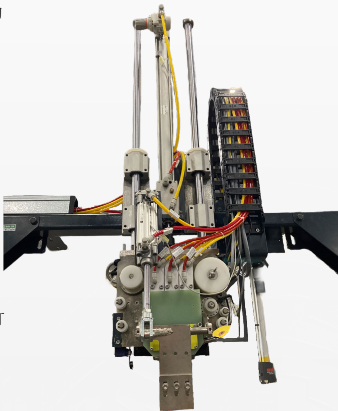
AkroMARK™ 上部打标器组件
